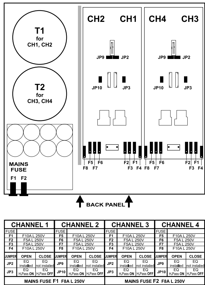
Abbildung 3.21: 4X DUAL Serie - Jumper und Sicherungen
