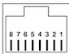
Abbildung 2.14: RS-485 Buchse
