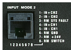
Abbildung 2.11: Multifunktionsanschluss
