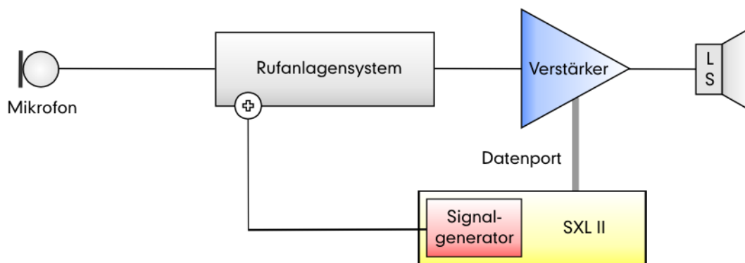
Abbildung 3.76: SXL II - Linienüberwachung
