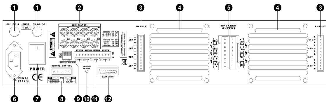
Abbildung 3.23: 8X Serie - Rückansicht
