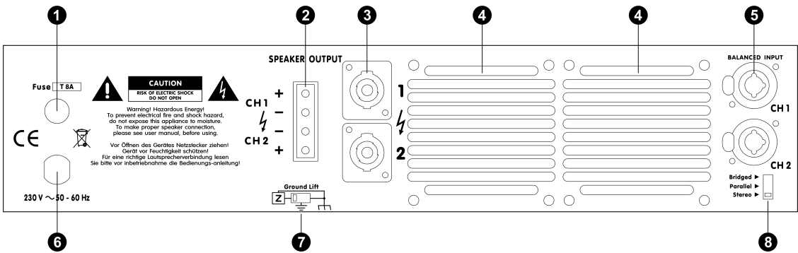
Abbildung 3.2: BASIC Serie - Rückansicht
