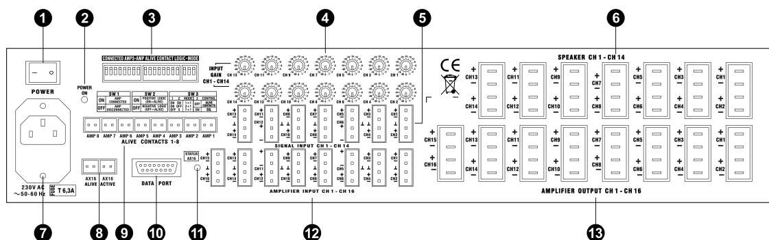
Abbildung 3.40: AX16 - Rückansicht
