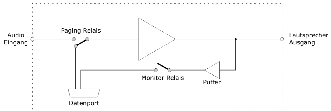
Abbildung 3.9: XR Serie - Pflichtrufeingang und Monitorausgang
