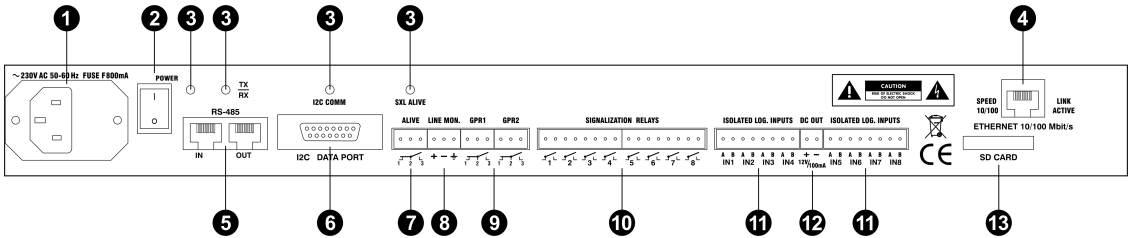
Abbildung 3.56: SXL II - Rückansicht
