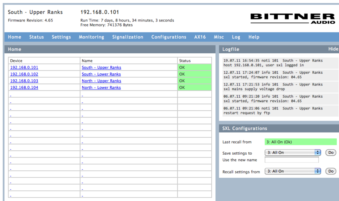
Abbildung 3.67: SXL II - Webinterface
