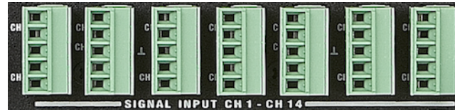
Abbildung 3.45: AX16 - Signaleingänge
