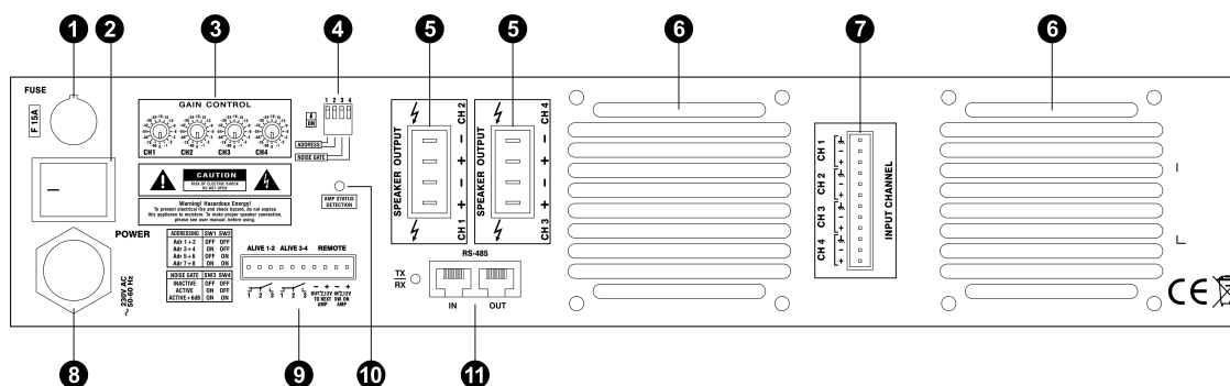
Abbildung 3.11: 4X Serie - Rückansicht
