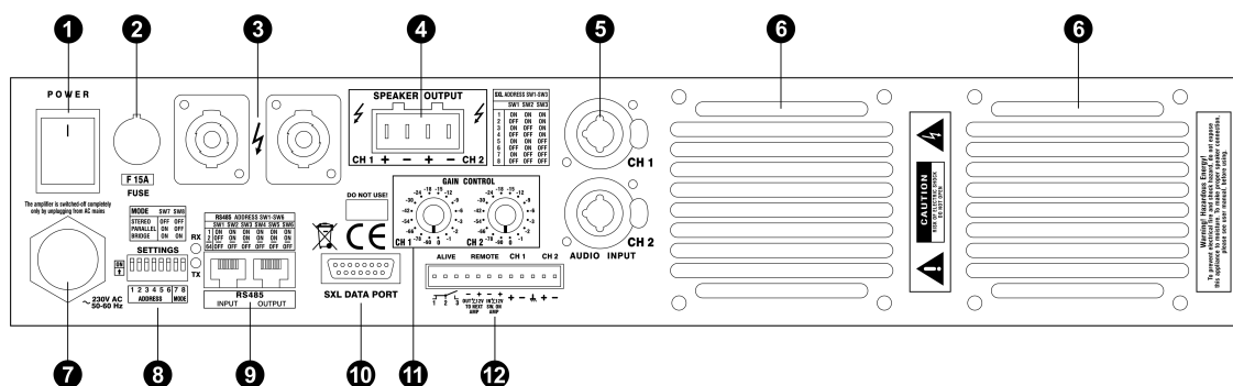
Abbildung 3.7: XR Serie - Rückansicht
