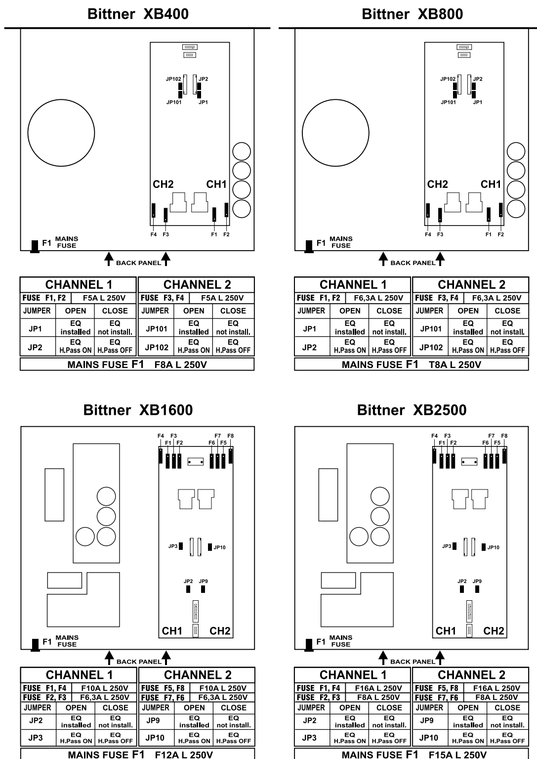
Abbildung 3.5: XB Serie - Jumper und Sicherungen
