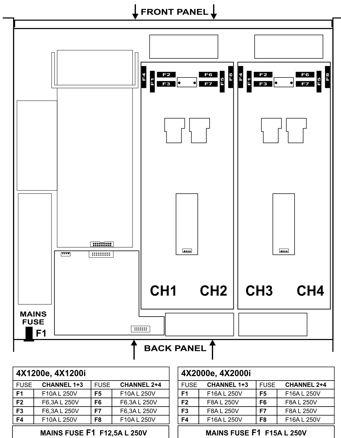
Abbildung 3.17: 4Xi/4Xe Serie - Sicherungen
