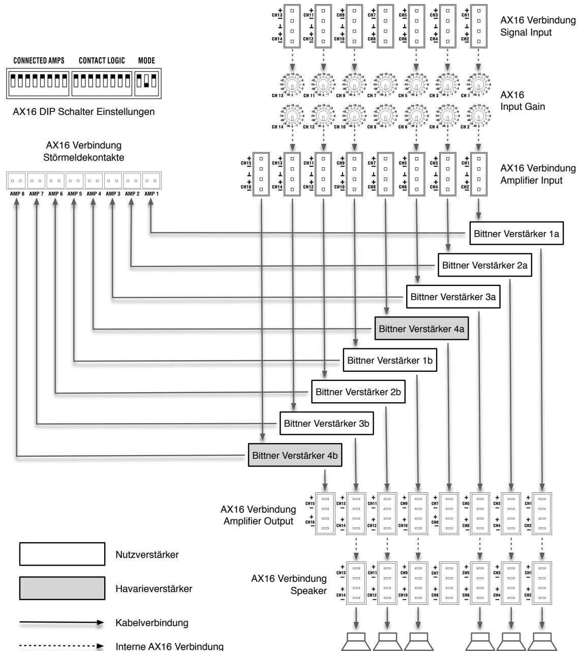
Abbildung 3.54: AX16 - Variante 3+1 mit 4-Kanal Verstärkern und Störmeldekontakten
