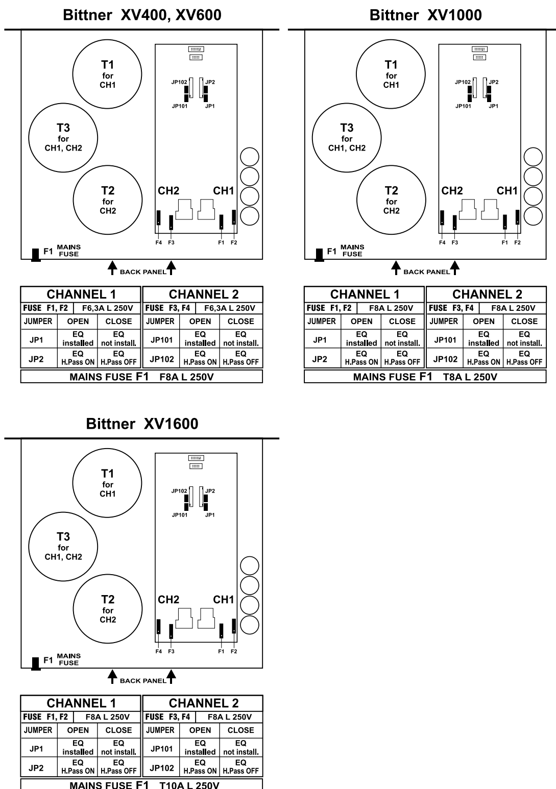
Abbildung 3.27: XV Serie - Jumper und Sicherungen
