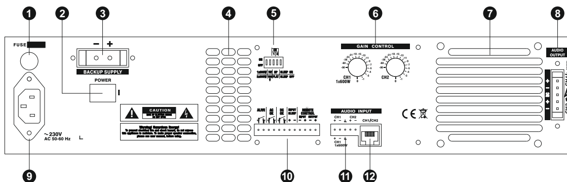
Abbildung 3.32: 2DXV Serie - Rückansicht
