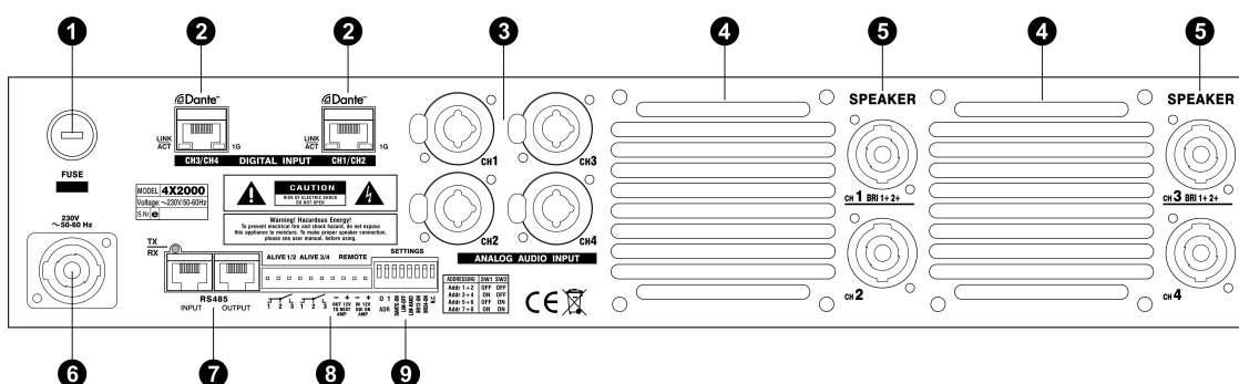
Abbildung 3.16: 4Xe Serie - Rückansicht
