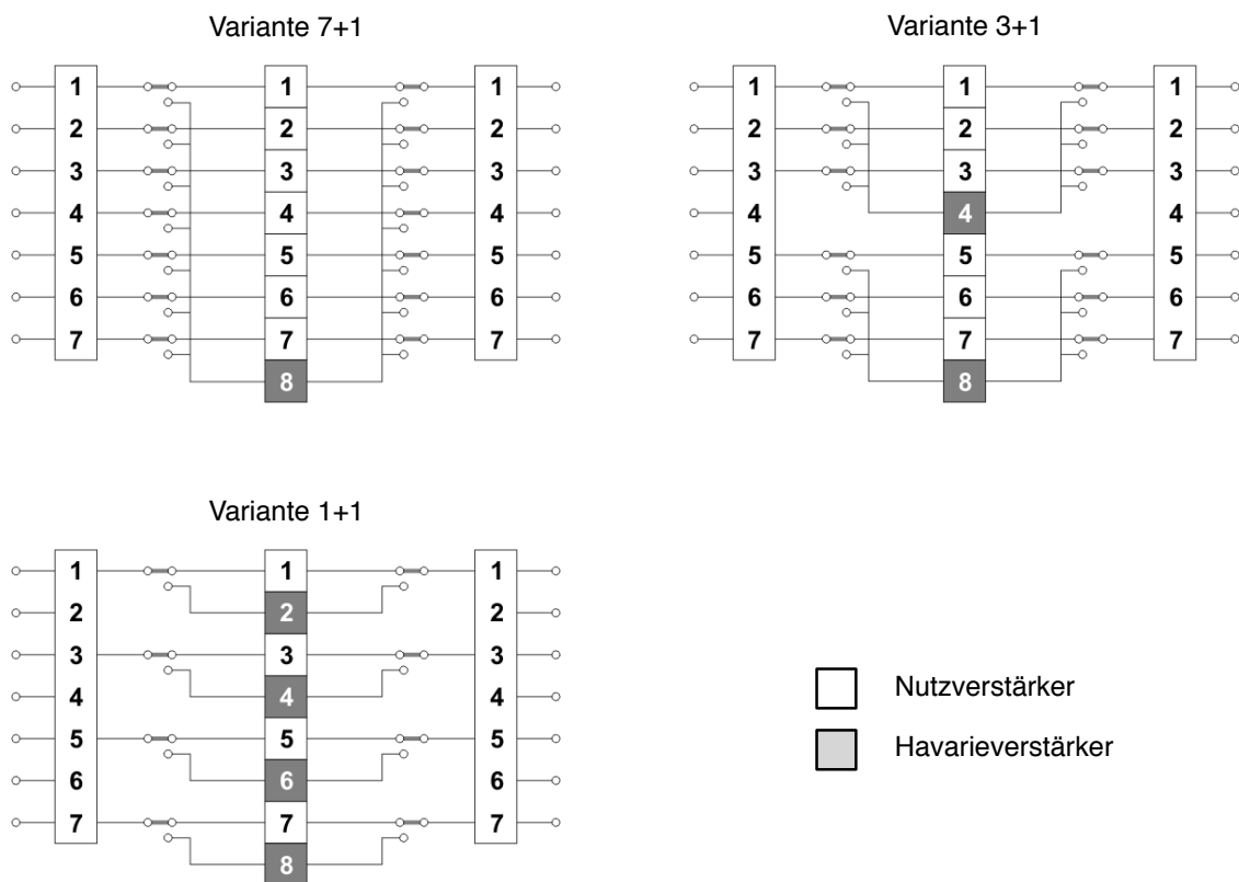
Abbildung 3.44: AX16 - Umschaltvarianten
