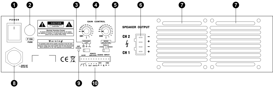
Abbildung 3.4: XB Serie - Rückansicht
