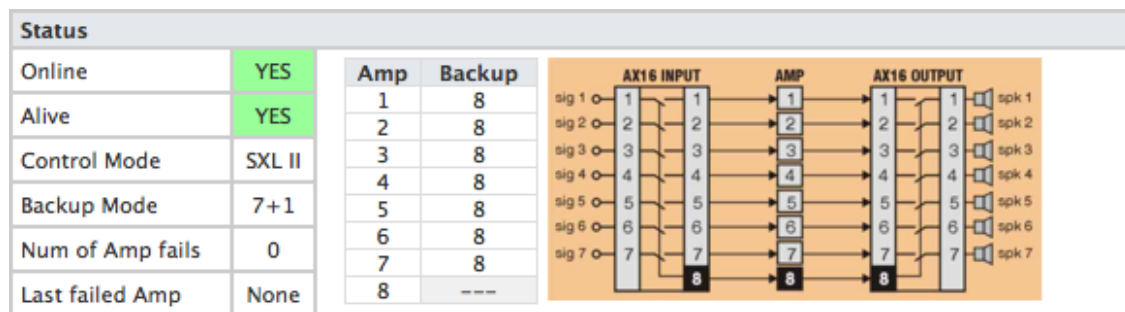
Abbildung 3.75: SXL II - Webinterface: Statusinformationen
