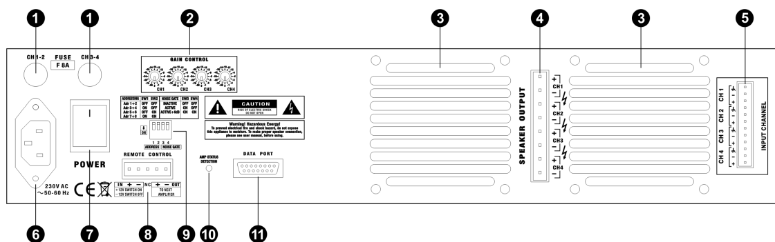
Abbildung 3.20: 4X DUAL Serie - Rückansicht
