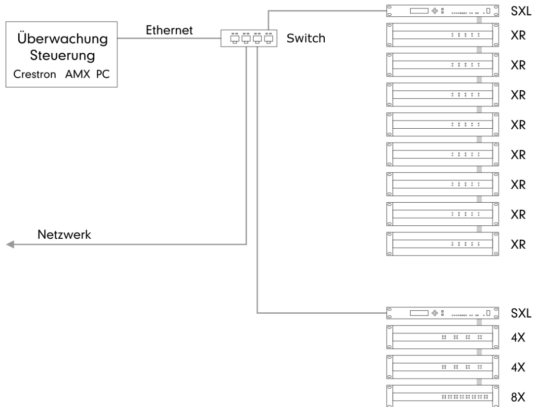
Abbildung 3.57: SXL II - Einbindung in ein Ethernet-Netzwerk
