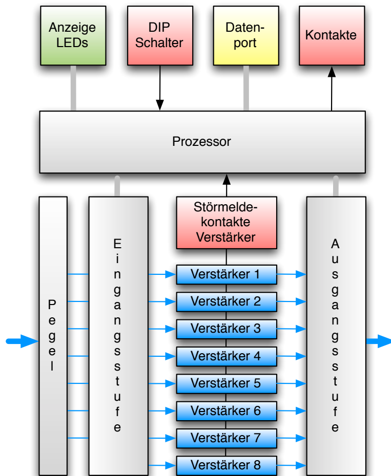
Abbildung 3.38: AX16 - Block Diagramm
