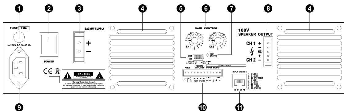
Abbildung 3.29: XV DC Serie - Rückansicht
