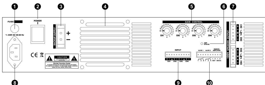
Abbildung 3.34: 4DXV Serie - Rückansicht
