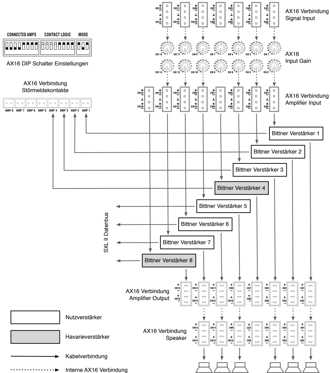
Abbildung 3.53: AX16 - Variante 3+1 mit SXL II und Störmeldekontakten
