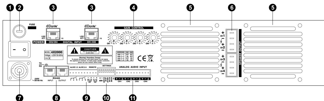
Abbildung 3.14: 4Xi Serie - Rückansicht
