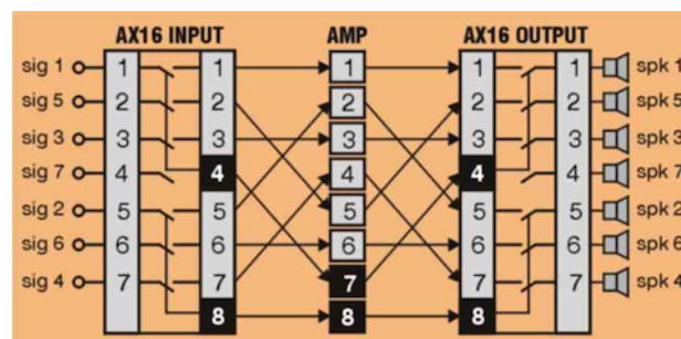
Abbildung 3.77: SXL II - Kreuzverkabelung für 4X/8X Betrieb
