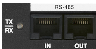
Abbildung 2.13: RS-485 Datenport
