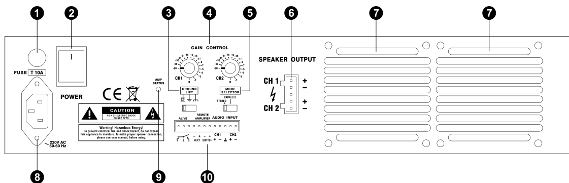
Abbildung 3.26: XV Serie - Rückansicht
